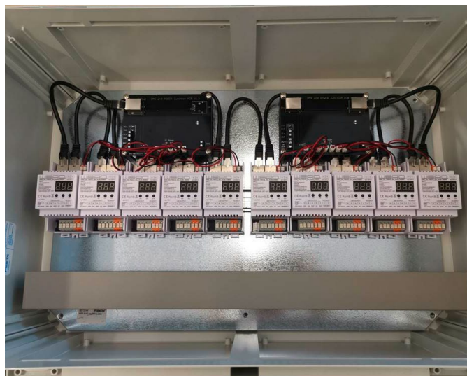
Abmessungen: LxBxH=600x400x210mm
